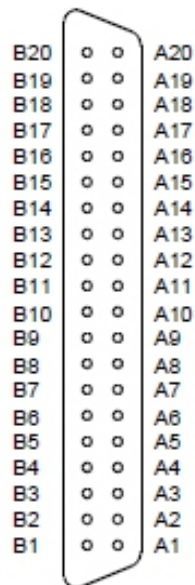
模組正視圖
