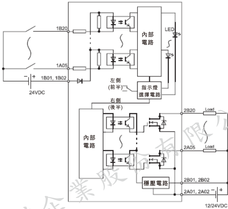
外部配線
