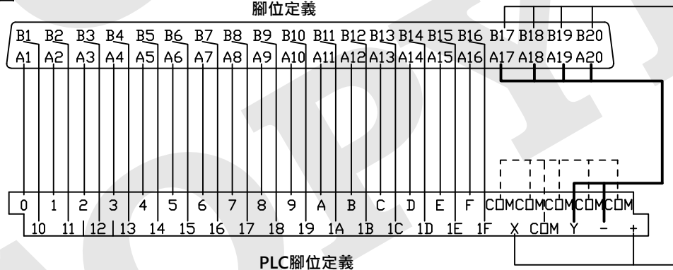
腳位圖：
