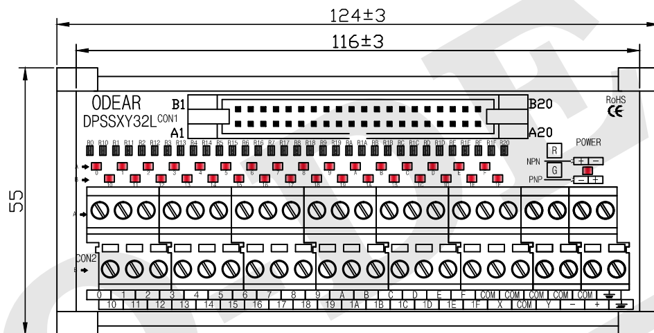
CONNECTOR 腳位定義
