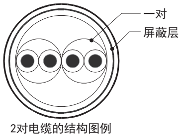
2对电缆的结构图例
