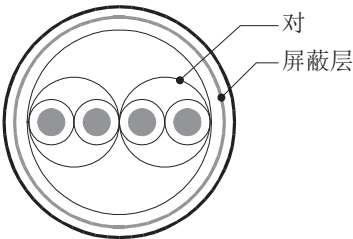
2对电缆的结构图示例
