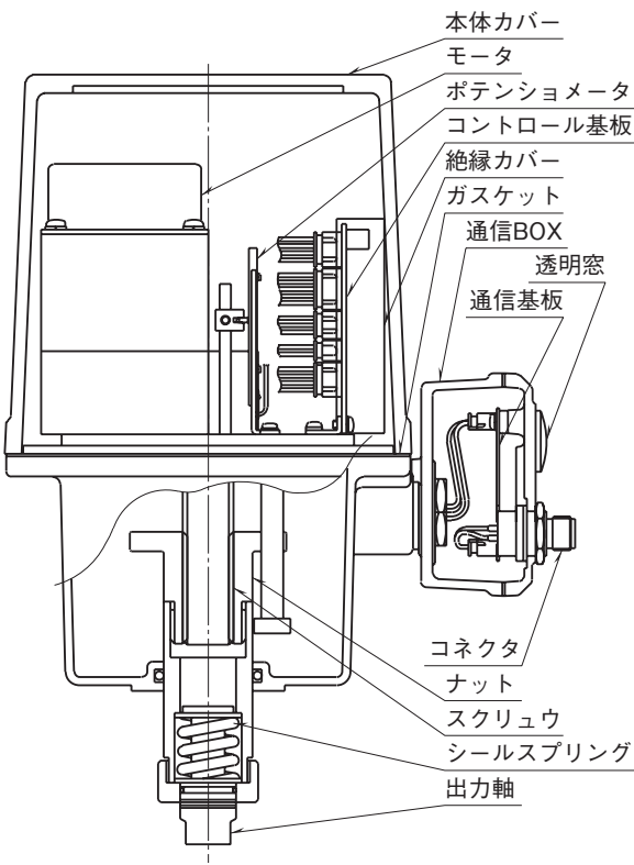
図2 各部の名称 (MSP6D)
