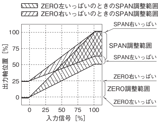
図5 入出力特性（調整範囲）
