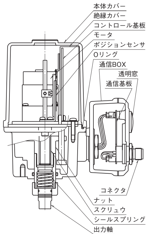
図1 各部の名称 (MSP4D、MSP5D) 注) MSP4D は一部構造が異なります。
