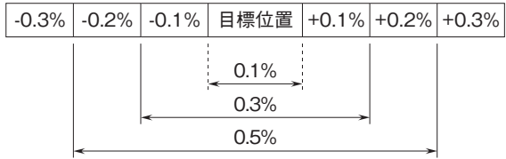
図9 DeadBand（不感帯幅）の推移
