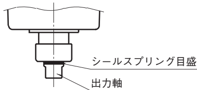
図 8 シールスプリング
