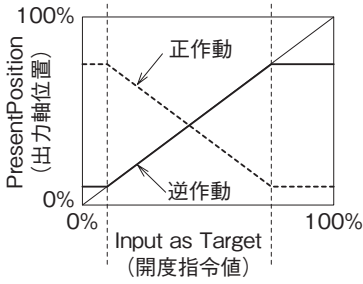
図12 入力リミッタ
