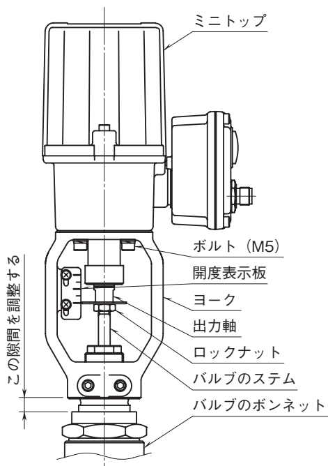
図 7 バルブへの取付例
