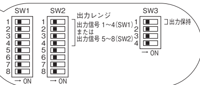
各種設定用ディップスイッチ
