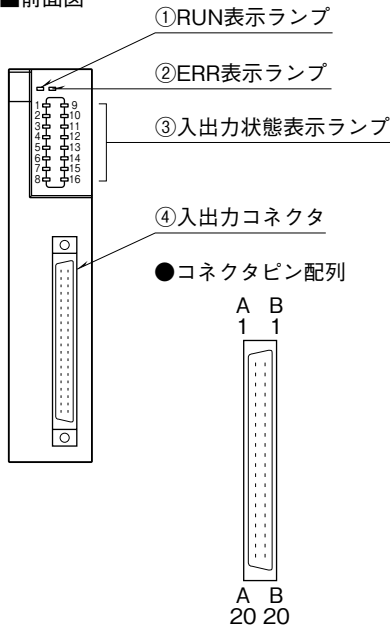
■前面図
