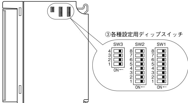
■側面図
