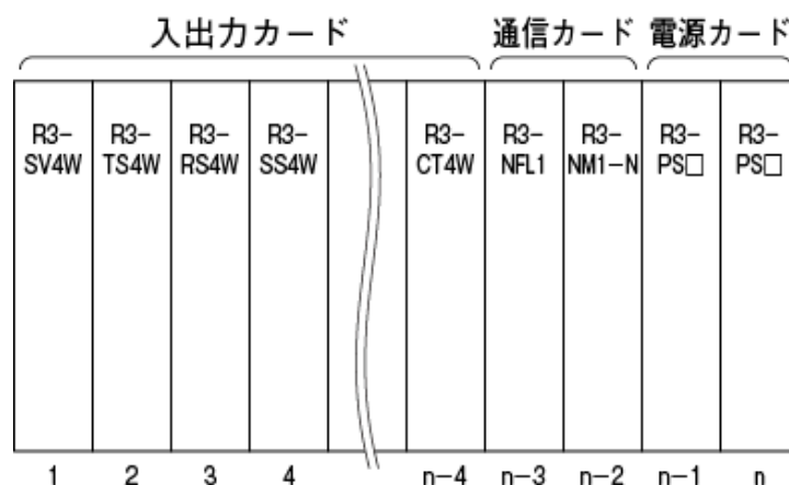
図 4-1 カードの実装位置の例
