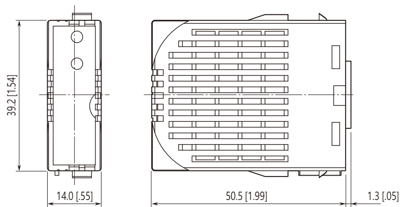
外型尺寸圖 單位: mm [inch]
