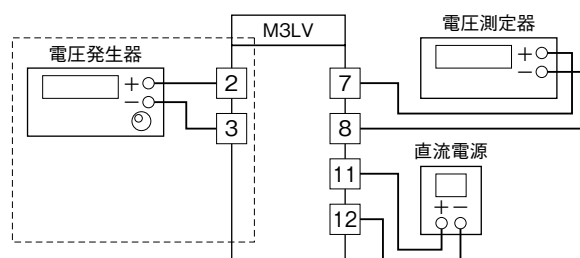
この接続例は電圧入力 (V) の場合を示します。 他の入力の場合は、端子接続図を参照して下さい。
