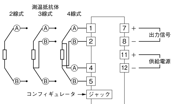
端子接続図
