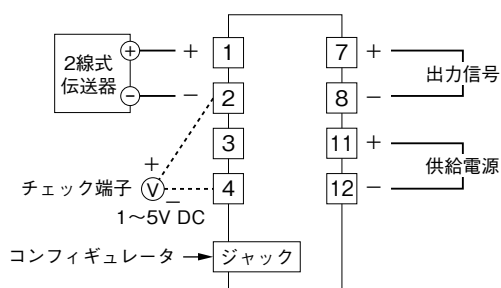
端子接続図
