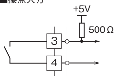
■接点入力
