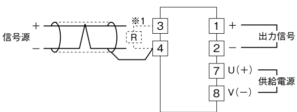
端子接続図
