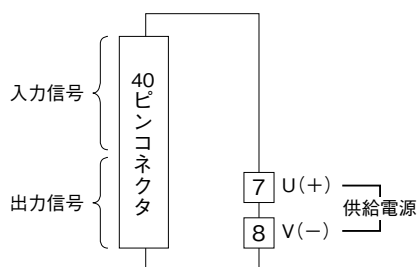
端子接続図
