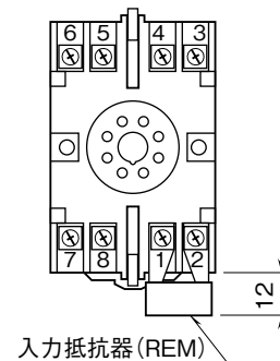
端子番号図 (単位 : mm)
