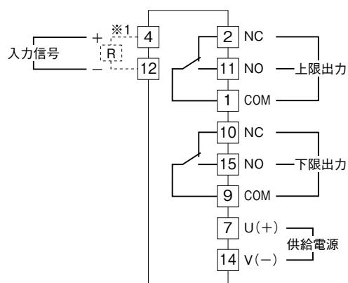
端子接続図
