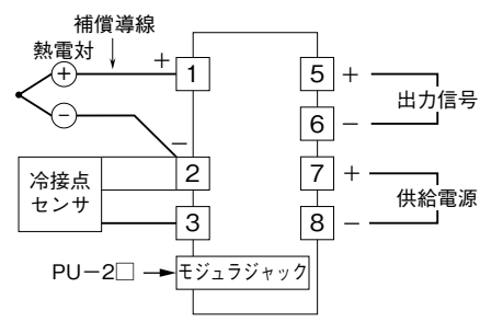
端子接続図
