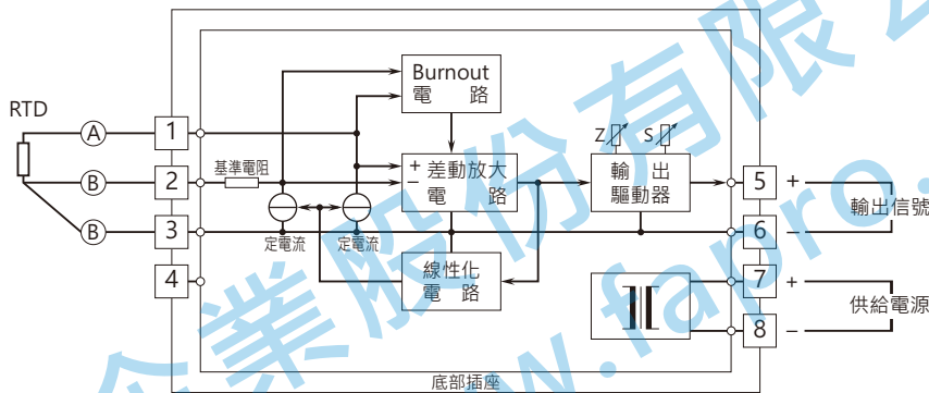
電路概要和接線圖
