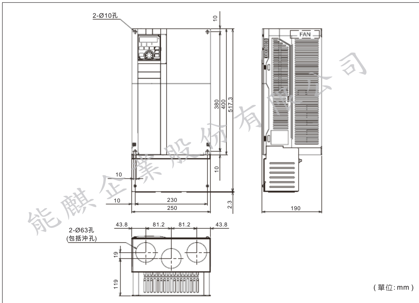
三菱電機FR-F820-00770-3-N6(18.5K)、00930-3-N6(22K)、01250-3-N6(30K)變頻器外型尺寸圖
