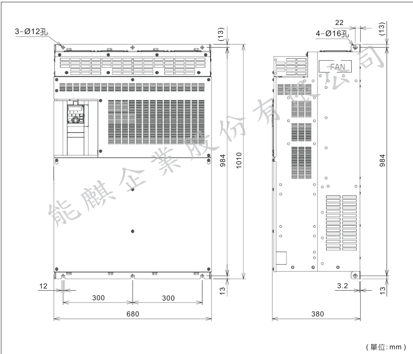
三菱電機FR-A840-05470-1-60、FR-A840-06100-1-60、FR-A840-06830-1-60變頻器外型尺寸圖
