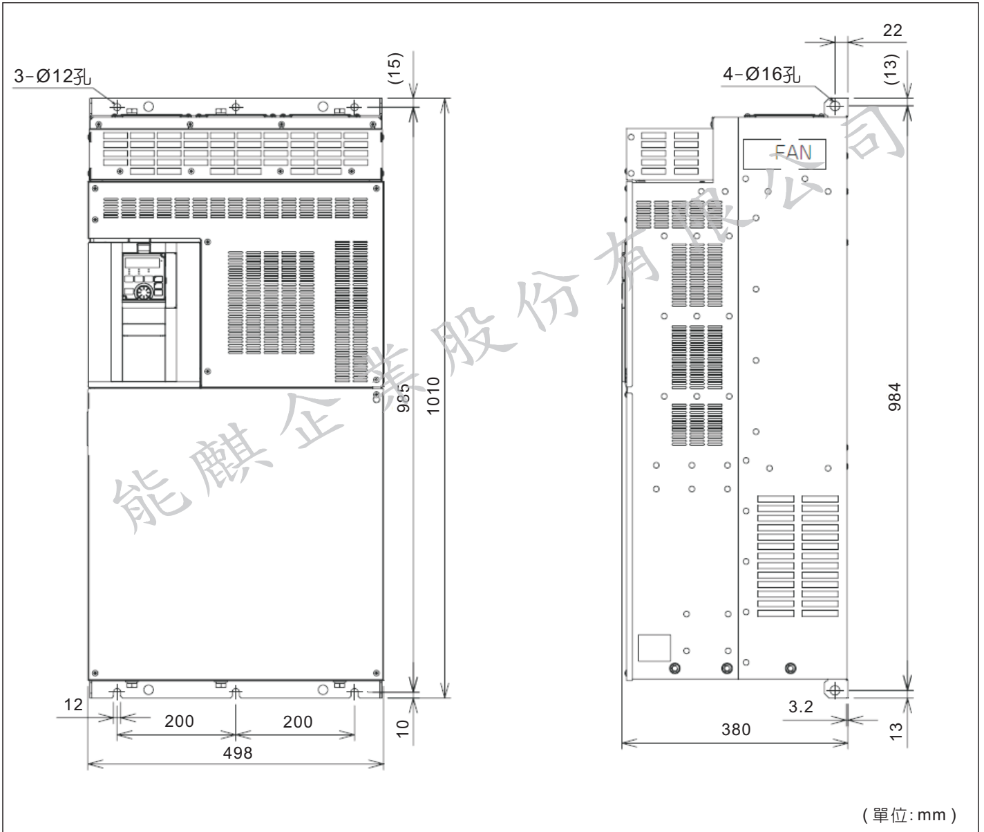
三菱電機FR-A840-04320-1-60、FR-A840-04810-1-60變頻器外型尺寸圖
