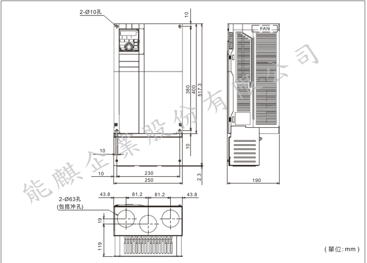
三菱電機FR-A840-00470-1-N6、FR-A840-00620-1-N6變頻器外型尺寸圖
