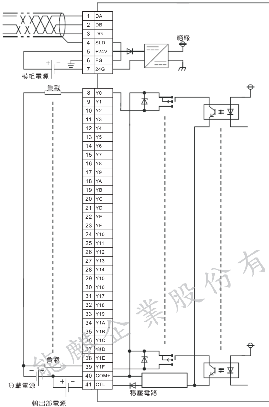
外部配線
